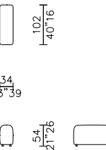
bracciolo - armrest 102
