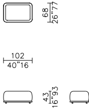
tavolo basso imbottito - padded low table 102
