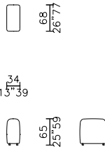
schienale - backrest 68
