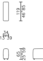
schienale - backrest 119
