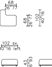
elemento MINI - unit MINI 102 L
