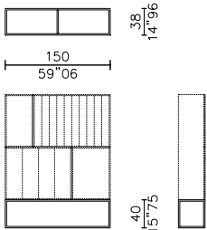
basamento - base *
